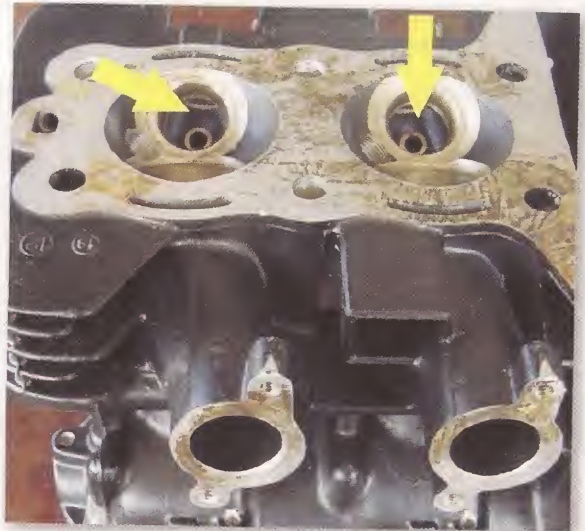
Detalles de las guías de la válvulas
